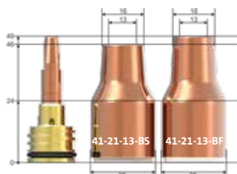
Gasdüse TEILE-NR. 41-21-13-BS 41-21-13-BF
